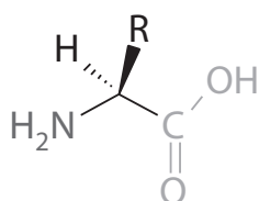
Slika 1. aminokiselina
