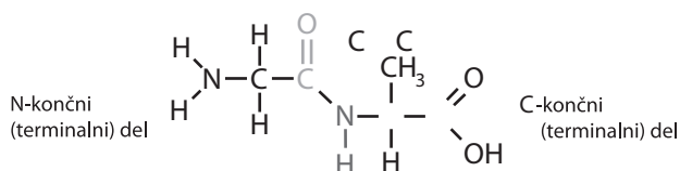
Slika 2. dipeptid
