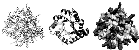
Slika 3. Strukture proteina
